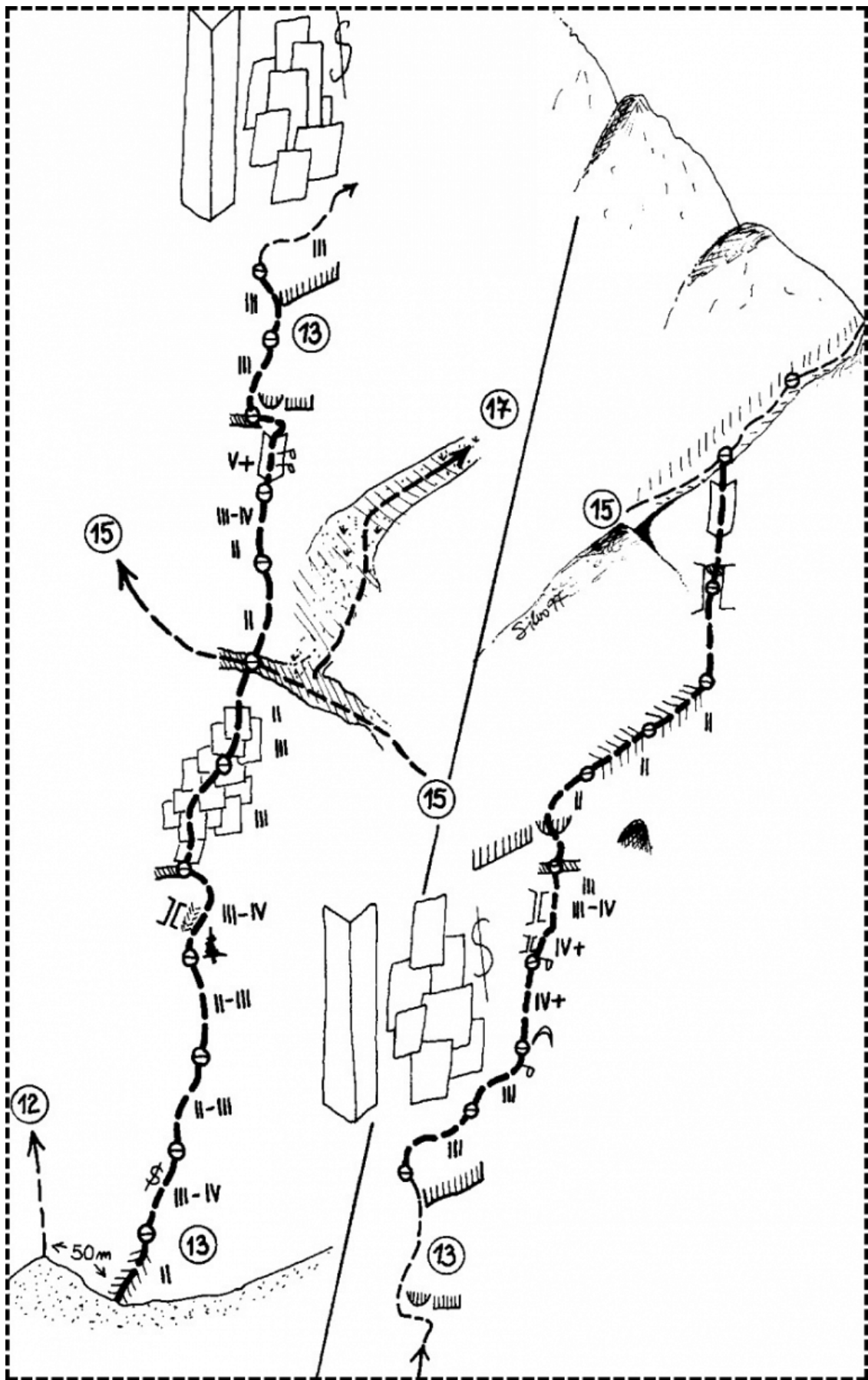
Planjava, severna stena: 12 Smer zadnjega srečanja, 13 Pepca, 15 Smer Gradišnik-Ogrin, 17 Celjska smer.
