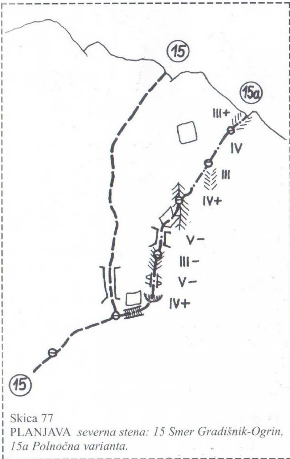
Planjava, severna stena: 15 Smer Gradišnik-Ogrin, 15a Polnočna varianta.
