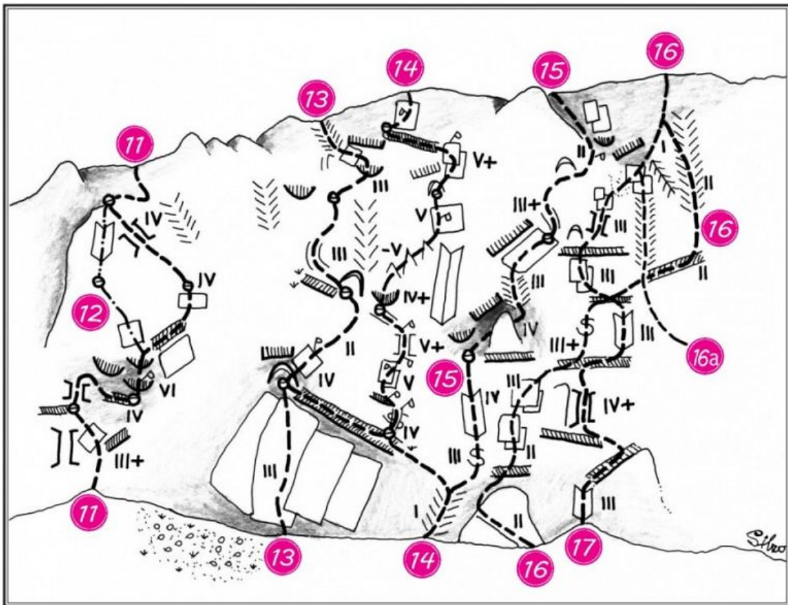
Vršiči, severozahodna stena: 11 Bela piramida, 12 Varianta Bele piramide, 13 Lepa smer, 14 Smer čez plošče, 15 Črna jama, 16 Smer PA, 16a Nežna, 17 Zavozlana smer.
